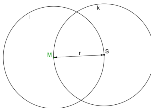
Fig. 15 Undersøgelse af parabler - trin 2
