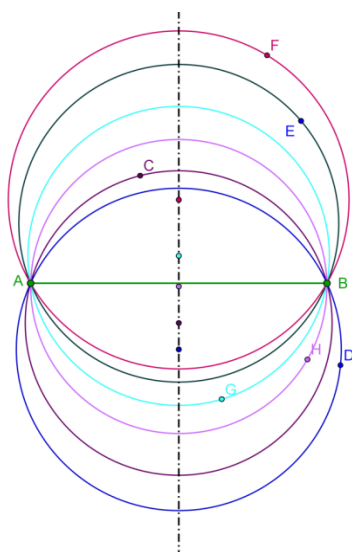
Fig. 8 Vinkelret halveringslinje, der er lavet i Geogebra
