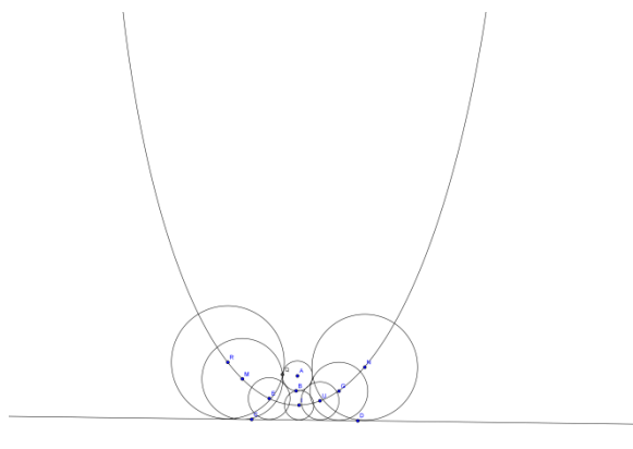
Fig. 12 Undersøgelse af parabler i Geogebra
