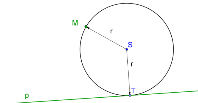
Fig. 16 Undersøgelse af paraboler - trin 3
