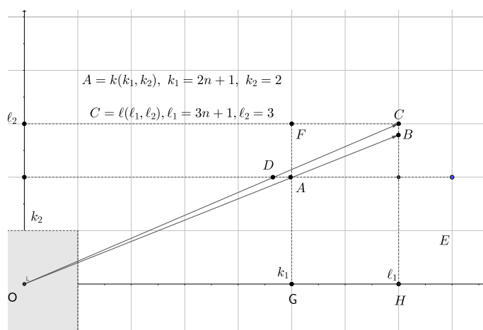
Figura 1: Il caso N \geq 3n + 1 .
